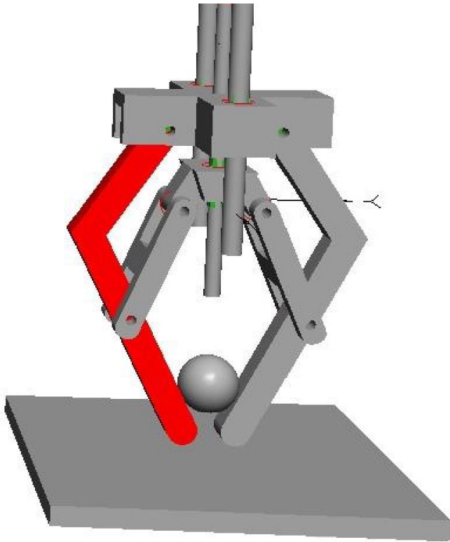
1. Chwytak - SimWise
