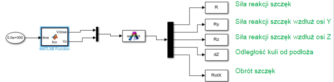
2. Symulacja SimWise + Simulink
